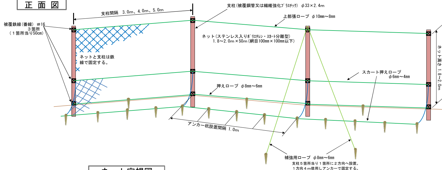
ネット定規図
