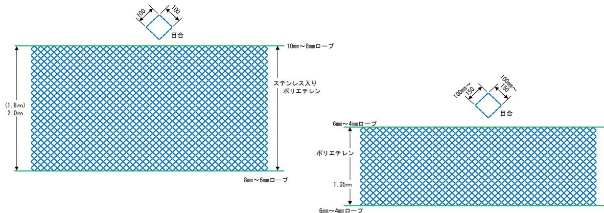
ネット定規図
