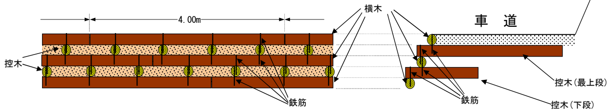
正面図 3段組
