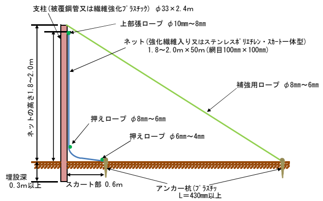
側面図
