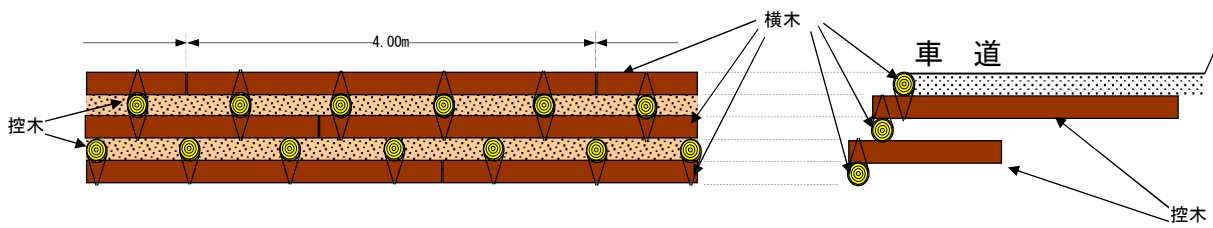
正面図 3段組
