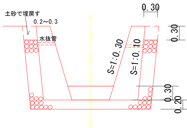
(ア) 標準断面図
