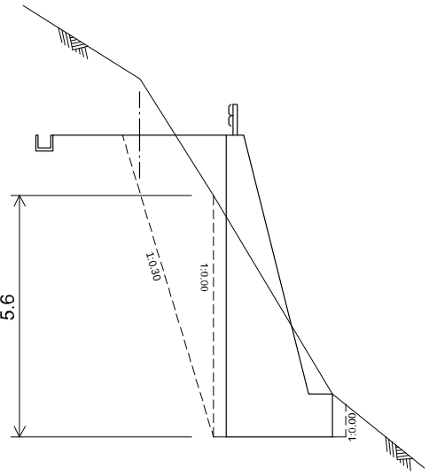
(6) 5.0m以上 (岩)
