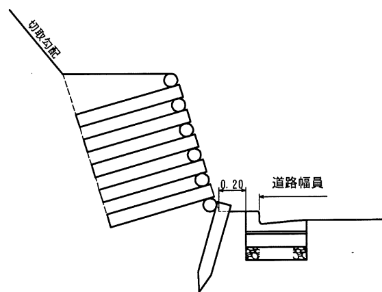
【丸太土留工】
