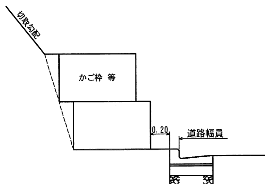
【かご枠等】
