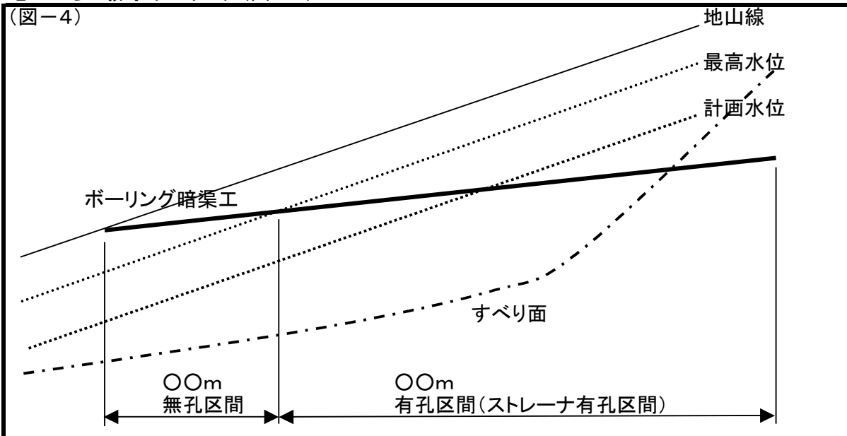
地上からの排水ボーリング(図-4)
