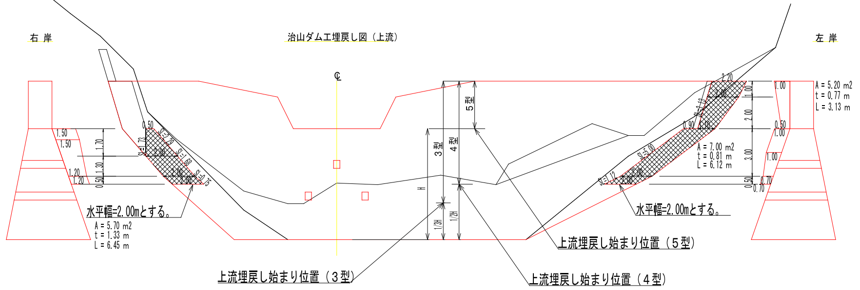
(3-2) 治山ダム工埋戻し図 (上流)
