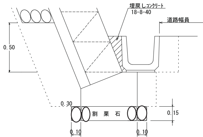
土 砂 基 礎
