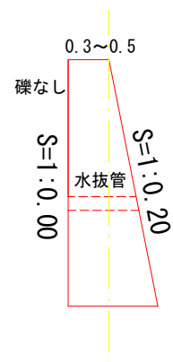
(ウ) 帯工
