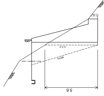
(6) 5.0m以上 (岩)
