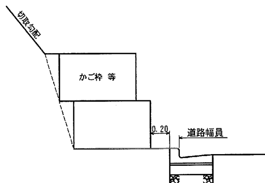
【かご枠等】
