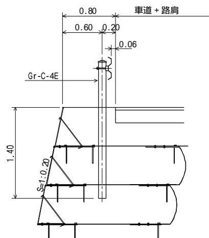
防護柵設置の詳細図
