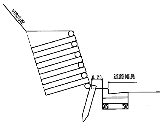
【丸太土留工】
