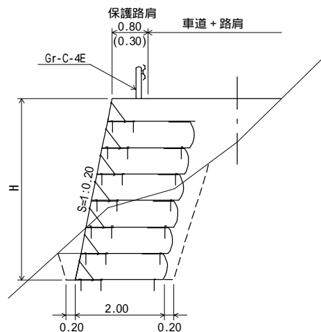
ジオバック工法の保護路肩幅
