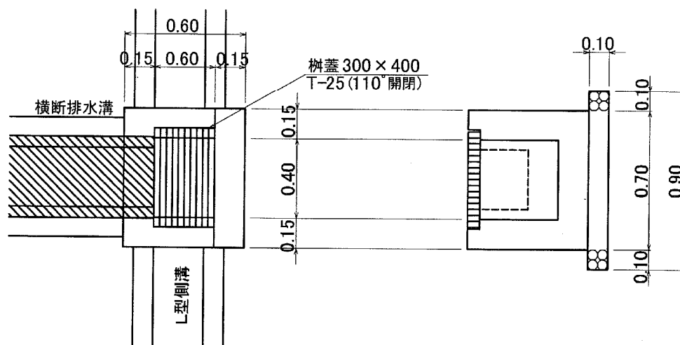
【平面図】
