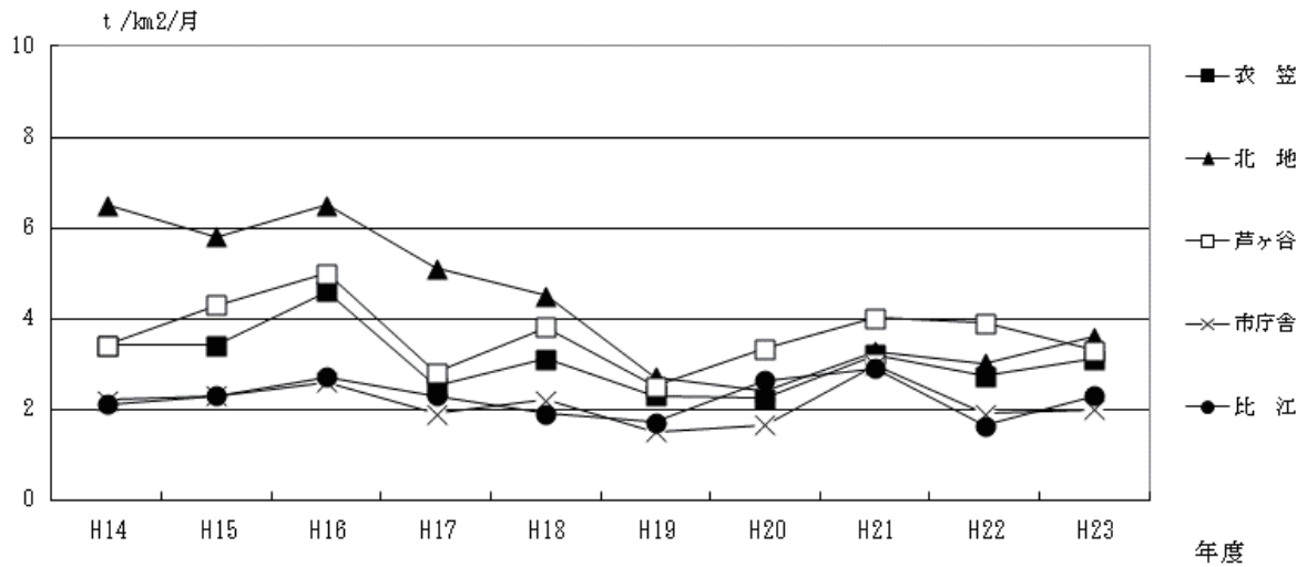
南国市の経年変化
