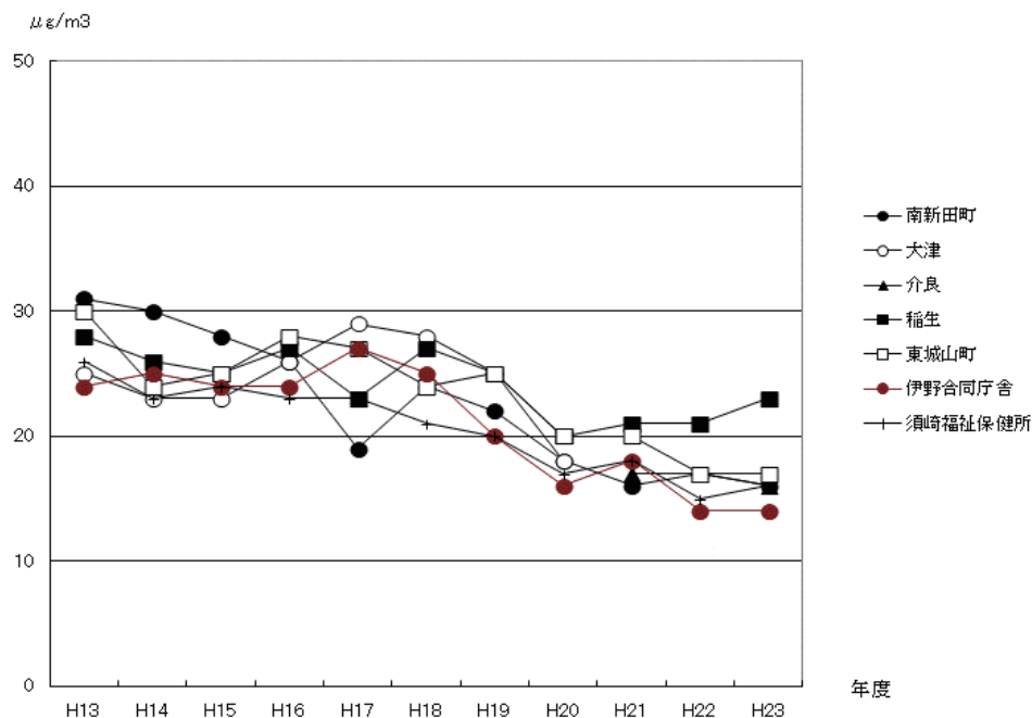
浮遊粒子状物質の経年変化
