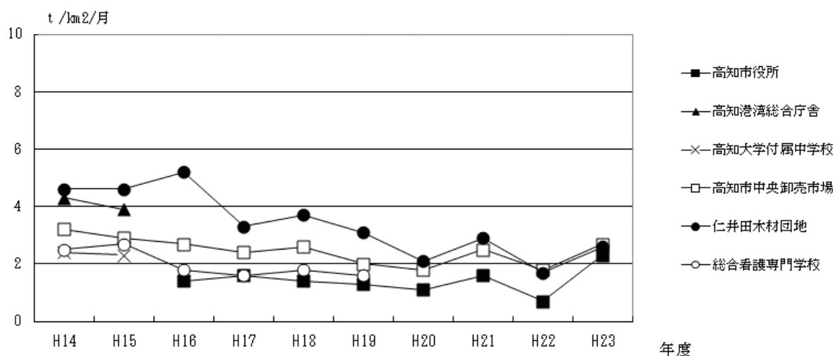
高知市の経年変化
