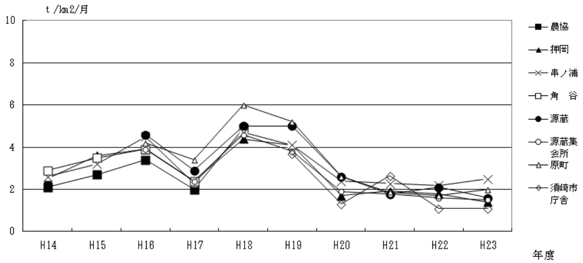
須崎市の経年変化
