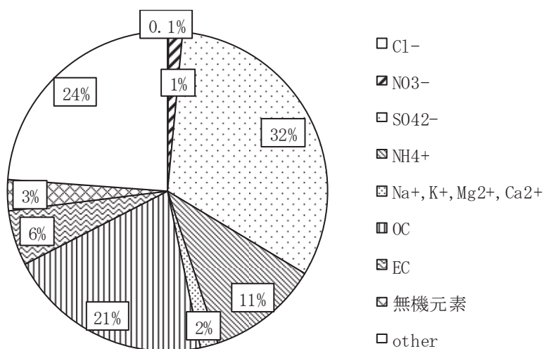
平成28年度成分割合（年平均）
