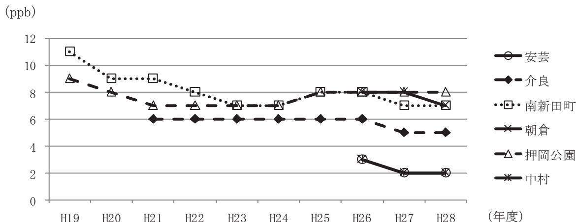
二酸化窒素年平均値の経年変化
