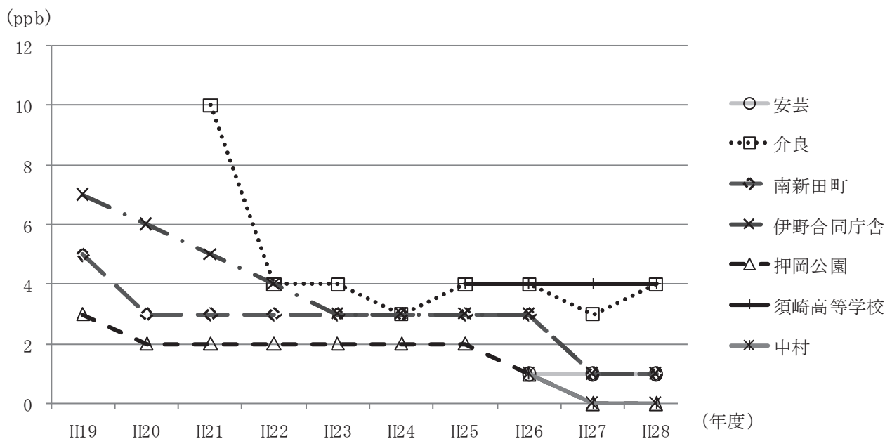
二酸化硫黄年平均値の経年変化
