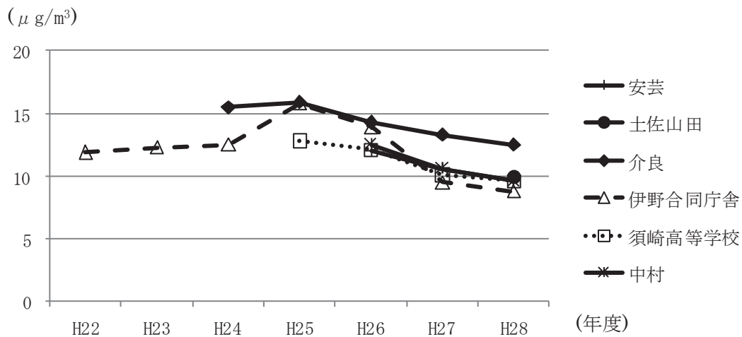
微小粒子状物質年平均値の経年変化
