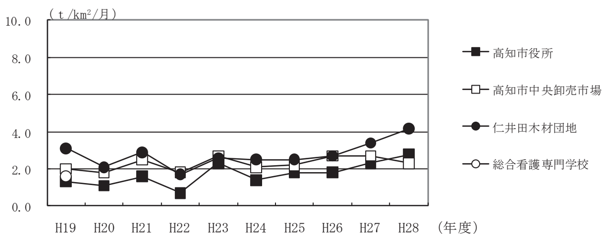
高知市の経年変化
