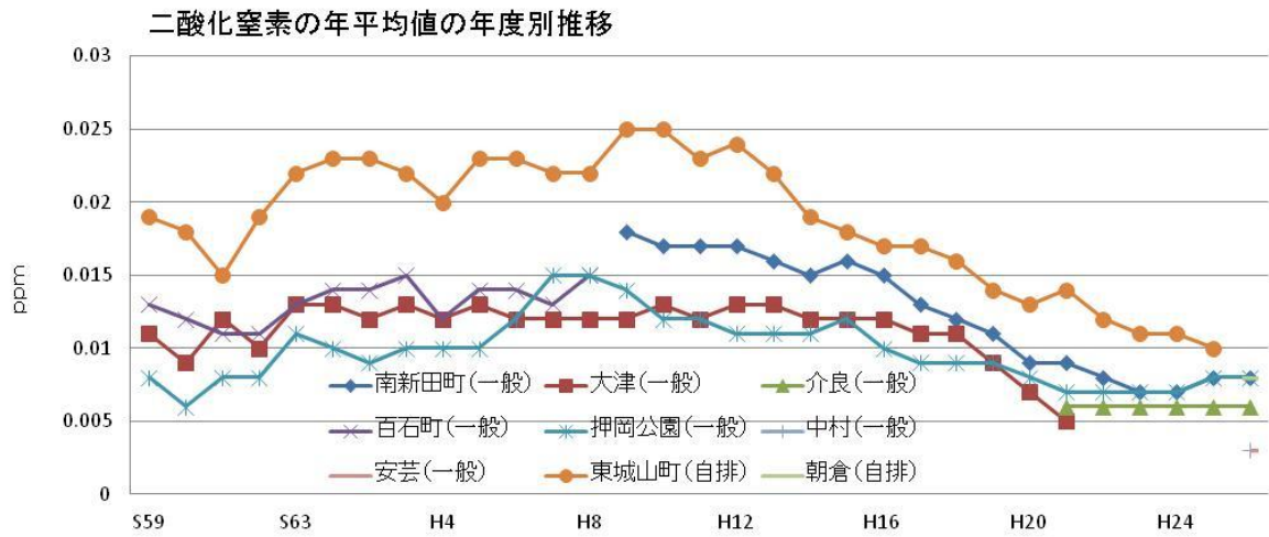
図2 二酸化窒素
