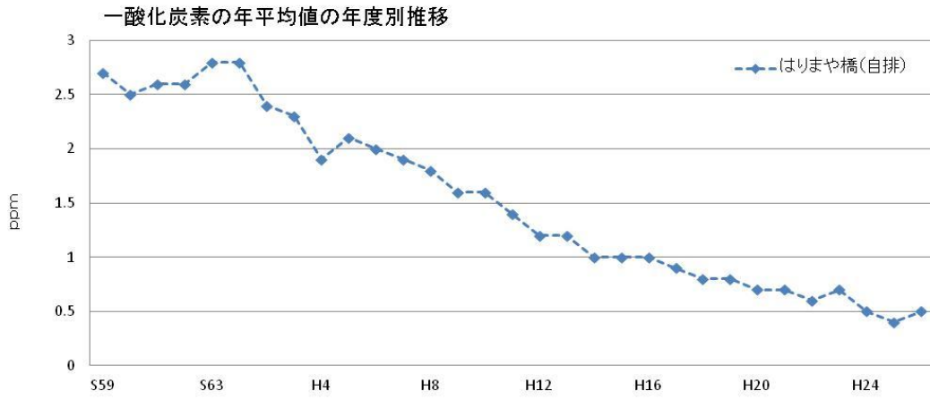
図5 一酸化炭素
