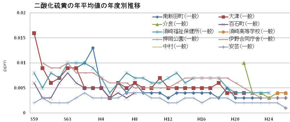
図1 二酸化硫黄
