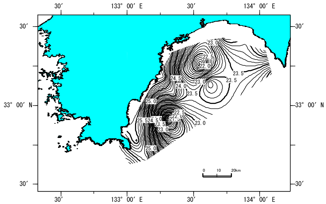
○深度 50m の水温分布
