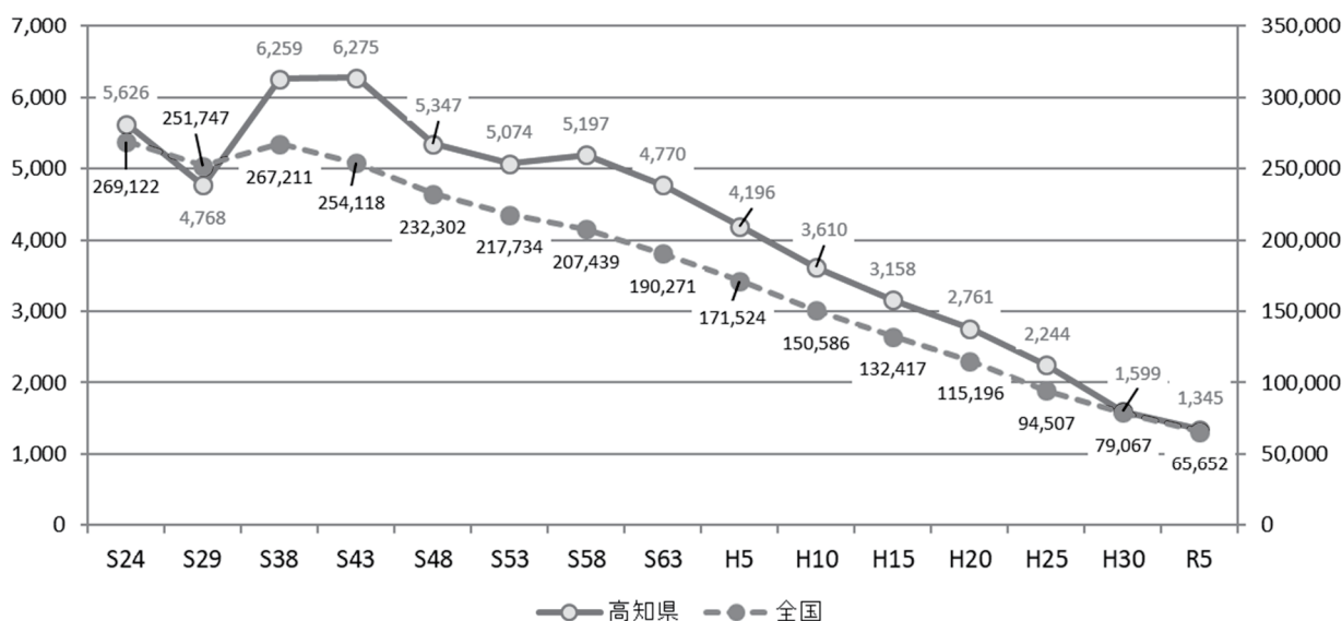
図表2 漁業経営体数の推移（高知県・全国）
