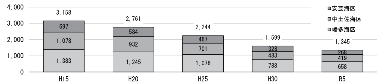
図表3 小海区別経営体数（高知県）
