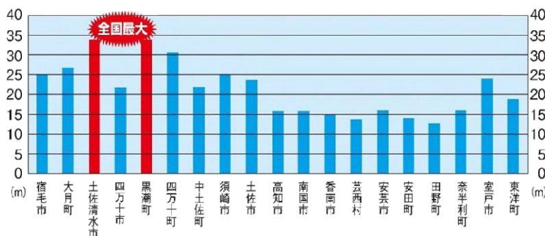
海岸線での津波の高さ
