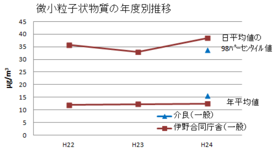
図6 微小粒子状物質
