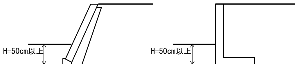
(a) 練ブロック積
