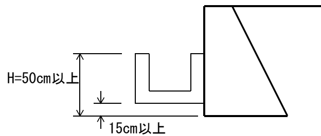
(d) 既存施設に隣接して設置する場合
