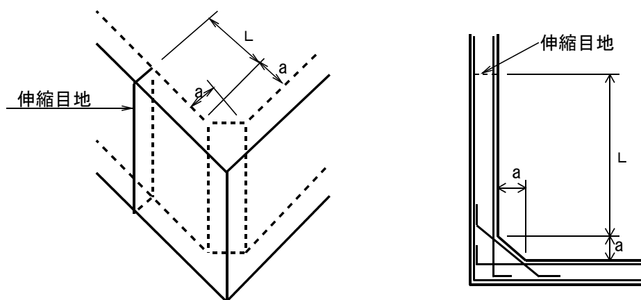
(a) 立体図
