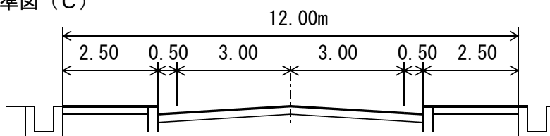
標準図 (C)
